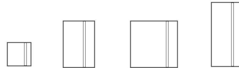
F128C/BAX140 ottone - brass F128C/MRX140 inox L 54 H 54 P 6 cm F128H/BAX180 ottone-brass F128H/MRX180 inox L 74 H 104 P 6 cm F128B/BAX210 ottone-brass F128B/MRX210 inox L 104 H 104 P 6 cm F128M/BAX290 ottone-brass F128M/MRX290 inox L 74 H 144 P 6 cm
